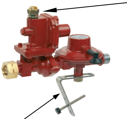
Abb. 11: Beispielhaftes Niederdruckregelgerät mit SAV und PRV (50 mbar, 4 kg/h) für Einfla-schenanlagen mit einem Füllgewicht von 33 kg sowie höhenverstellbarer Abstütz-vorrichtung
