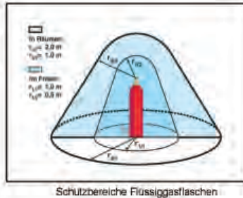
Schutzbereiche Flüssiggasflaschen
