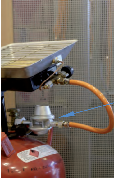
Abb. 25: Erforderliche Sicherheitseinrichtungen (hier: Druckregelgerät mit integrierter Überdrucksicherheitseinrichtung) für die Benutzung von Gasgeräten mit Schlauchleitungen bis maximal 0,4 m (Beispiel: Infrarotstrahler), Betrieb im Freien
