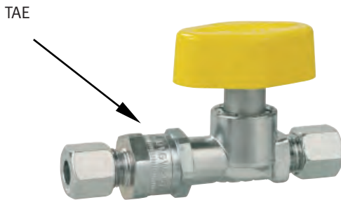
Abb. 24: Beispielhaftes Schnellschlussventil mit thermischer Absperreinrichtung (TAE)
