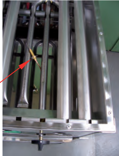
Abb. 29: Bräter mit am Brennerrohr anliegender Züandsicherung
