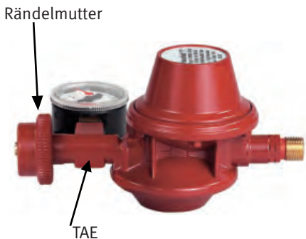
Abb. 23: Beispielhaftes Druckregelgerät mit integrierter Überdrucksicherheitseinrichtung und thermischer Absperrrichtung (TAE)
